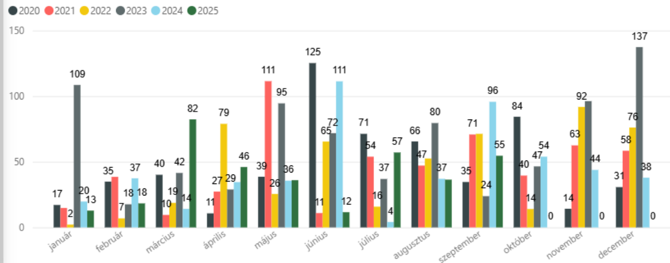
Havi csapadékmennyiség (mm)
