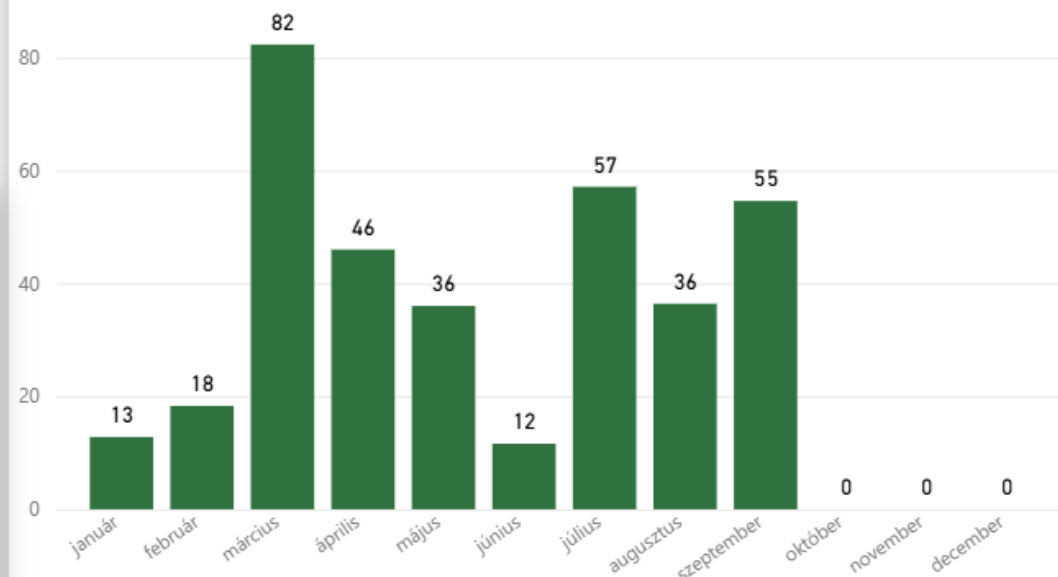
Havi csapadékmennyiség (mm)
